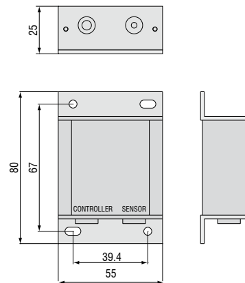
CP6001 kapazitiver Vorverstärker
