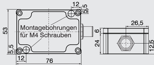
Abb. 2 Maßzeichnung, Abmessungen in mm, nicht maßstabsgetreu
