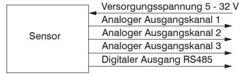
Abb. 4 Strom- und Spannungsausgang
