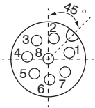
Abb. 3 Ansicht der Lötseite, 8-polig, A-kodiert, Buchse
